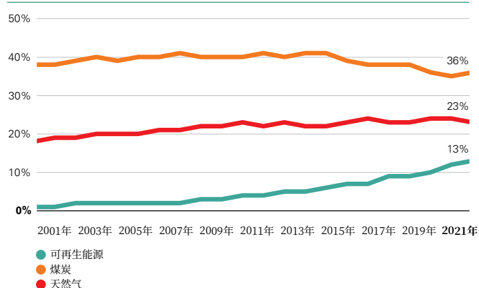
可再生能源在全球发电总量中的份额持续增加
